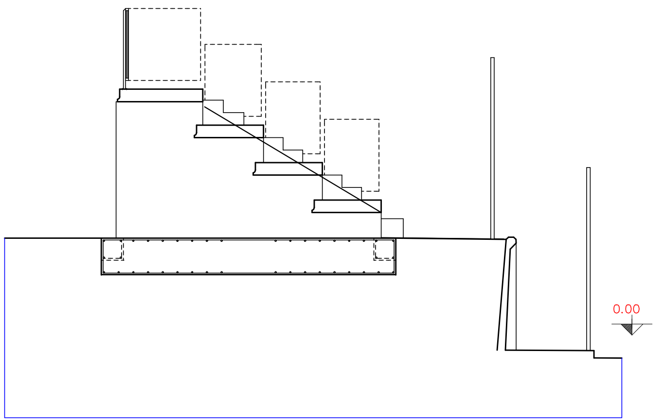
SEZIONE B-B TRIBUNE
