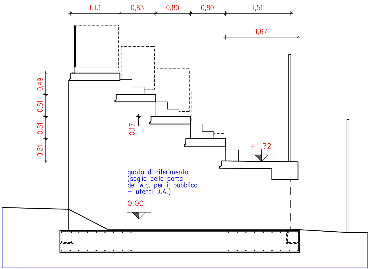
SEZIONE A-A TRIBUNE
