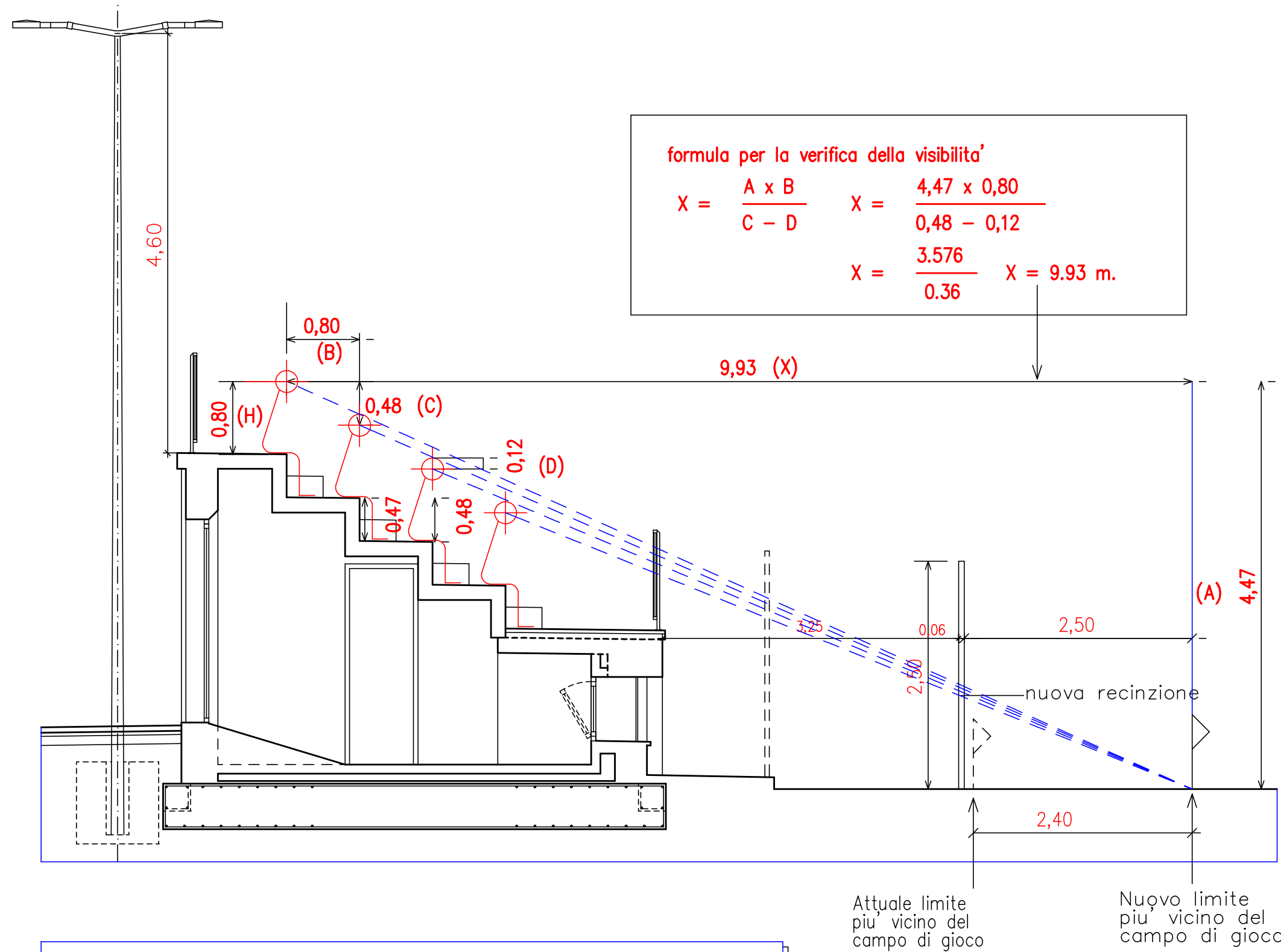
SEZIONE A-A TRIBUNE - VERIFICA DELLA VISIBILITA'
